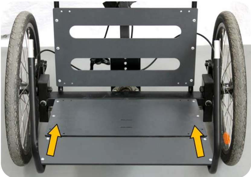
Abbildung 5 - Einführung der unteren Vorderrohre in die Ladefläche
