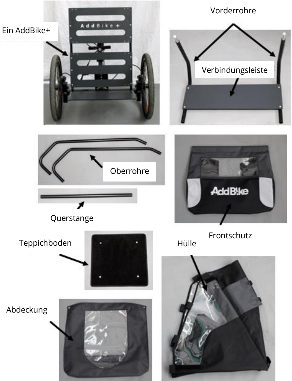
Abbildung 1 - Lexikon des Carry'Dog-Moduls
