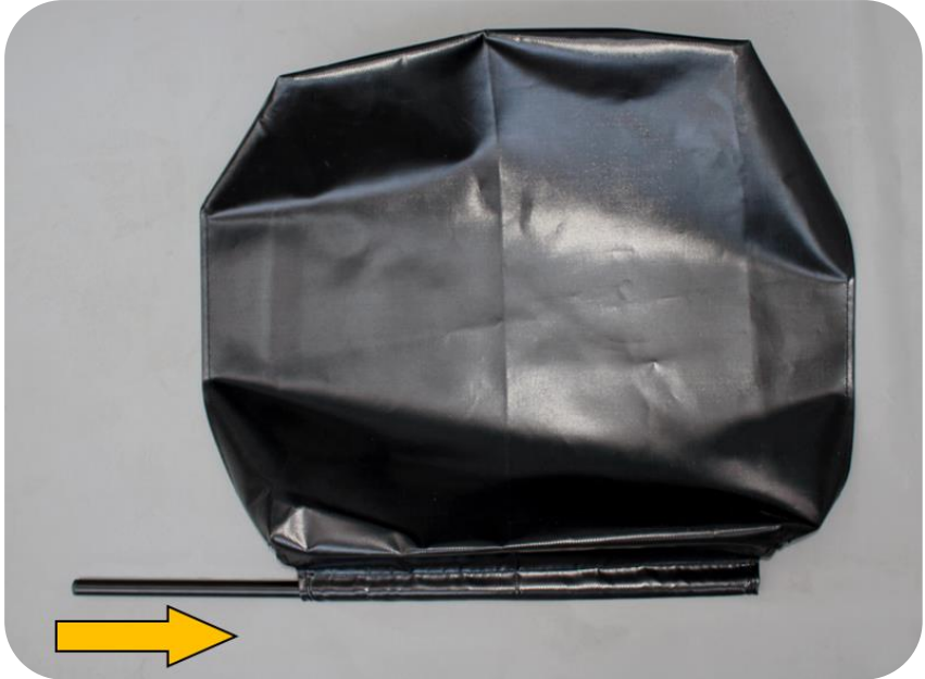
Abbildung 12 - Einführen der Querstange in den Überzug des Textilteils
