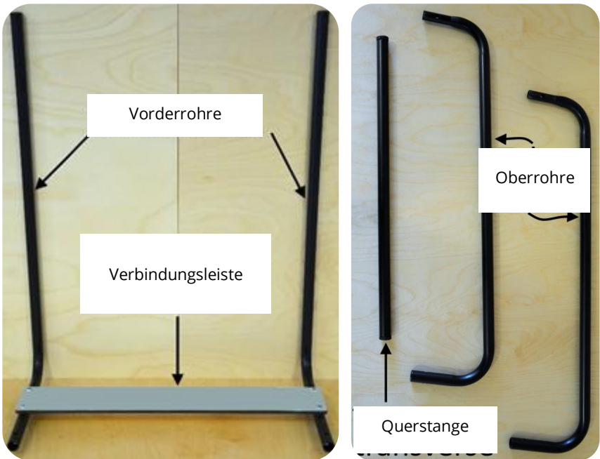
Abbildung 1 - Lexikon des Carry'Box-Moduls
