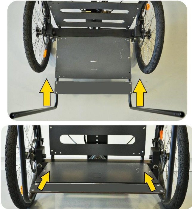
Abbildung 5 - Einführen der unteren Rohre in die Sitzfläche
