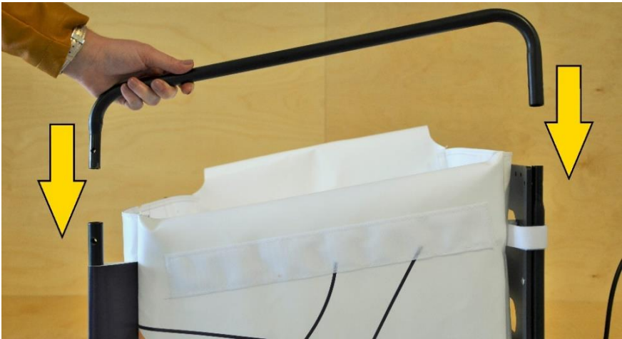
Figure 10 - Insertion des tubes haut dans le dossier
