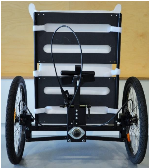
Figure 8 – Accroche de l'arrière du textile
