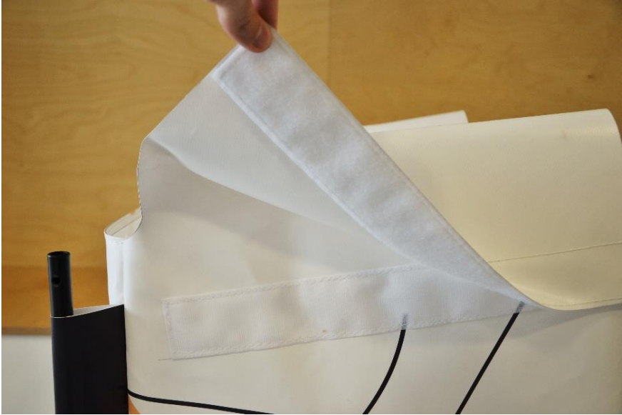
Figure 9 – Bande de textile à défaire
